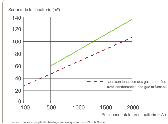
SURFACE DE LA CHAUFFERIE EN FONCTION DE SA PUISSANCE
