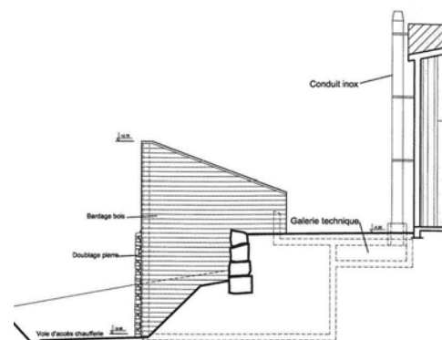
Chaufferie Base Sapeurs Saint Auban (06) Exemple d'implantation chaufferie + cheminée
